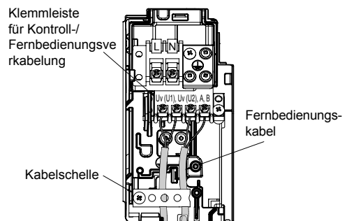
<Anschluss der Fernbedienungskabels>
