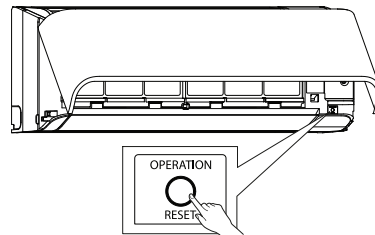
BETRIEBS-/RESET-TASTE
