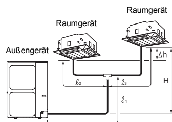
Abbildung simultaner Twin
