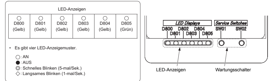
LED-Anzeigen-Anfangsstatus
