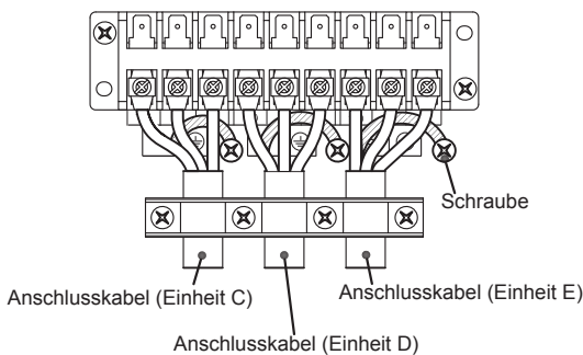
* Verbindungsbeispiel (RAS-5M34U2AVG-E)
