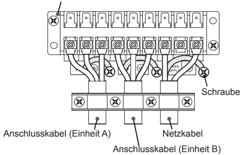
Verteilerblock (Verbindungskabel)
