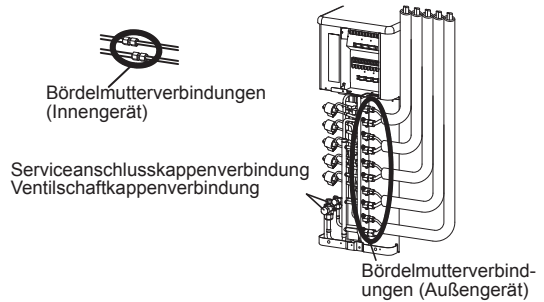
* Prüfpunkt-Beispiel (RAS-5M34U2AVG-E)
