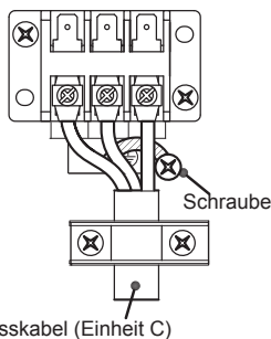
* Verbindungsbeispiel (RAS-3M26U2AVG-E)
