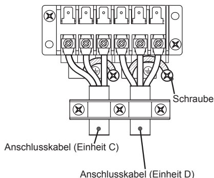
* Verbindungsbeispiel (RAS-4M27U2AVG-E)
