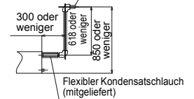
Abmessungen für Kondenswasserablauf nach oben
